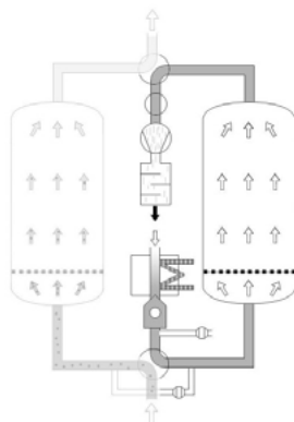
Lämmitysvaihe
