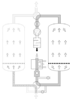
Jäähdytysvaihe
