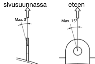
Kuljetus nosturilla
