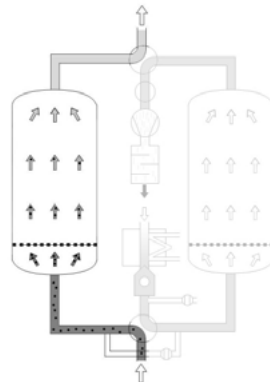
Adsorptio (tässä: absorptio vasemmassa säiliössä)
