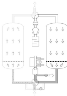
Paisuntavaihe
