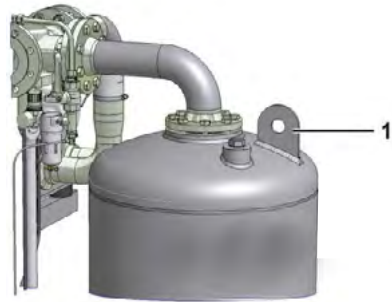
Nostosilmukat säiliössä
